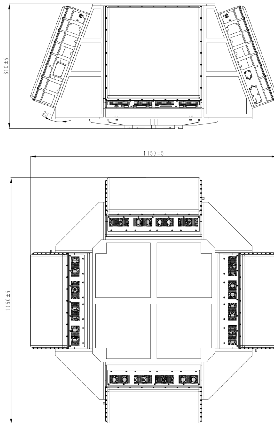
CR-PX16C 结构及安装尺寸图 (单位: mm)
